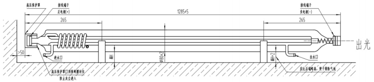
X2型激光管安装示意图
